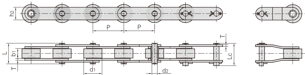
大滚子型 Large roller type
